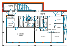
DOGRADNJA - PRIZEMLJE
